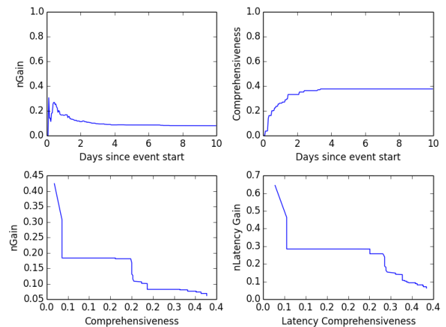
(d) Query 21
