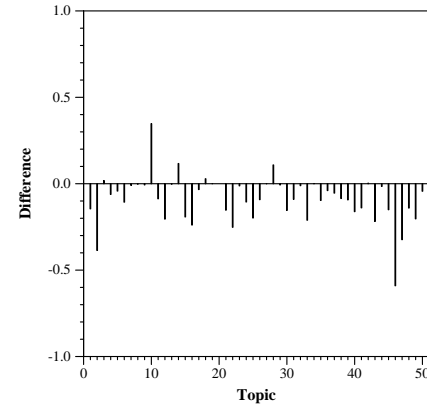
statAP Per Topic Median Diff, QUT.YUIR.2
