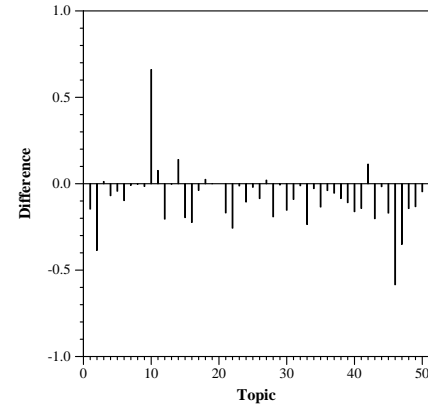
statAP Per Topic Median Diff, QUT.WatS.1
