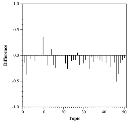
statAP Per Topic Median Diff, QUT.SIEL.1
