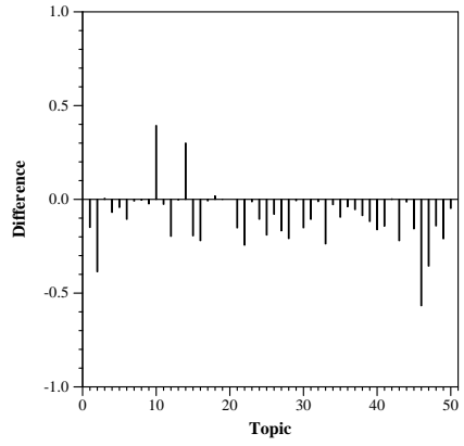
statAP Per Topic Median Diff, QUT.MSRC.2
